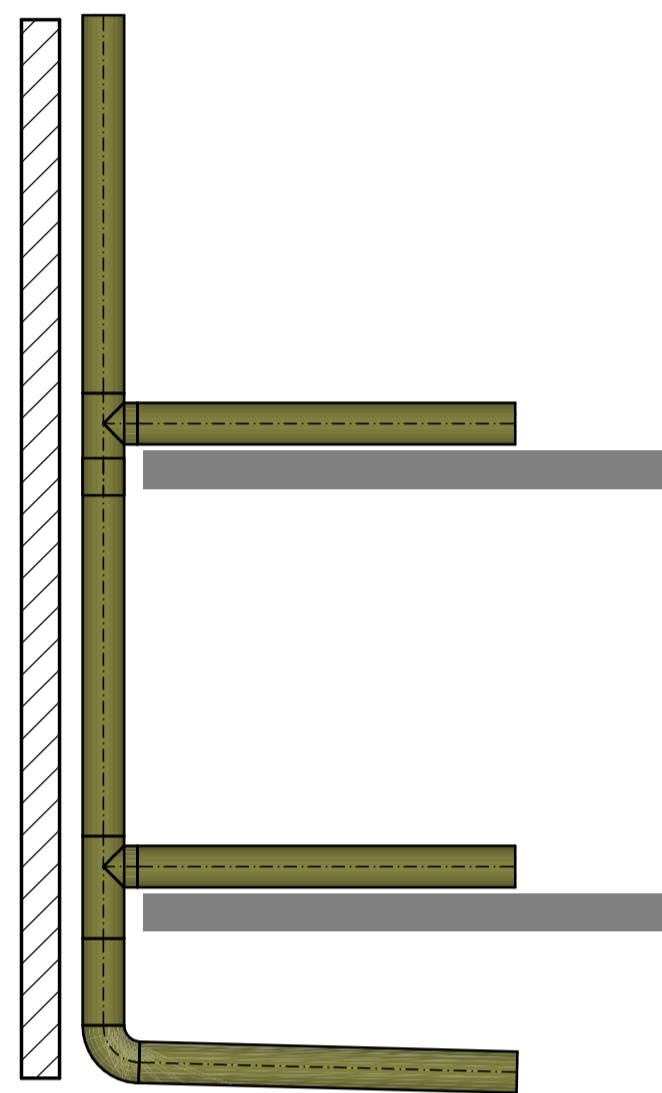
Umlenkung in liegende Leitung mit einem Bogen 88^\circ \pm 2^\circ
