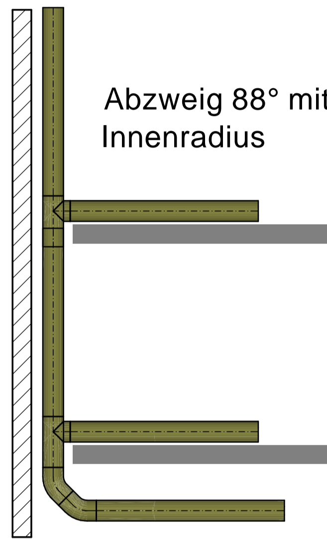
Umlenkung in liegende Leitung mit 2 Bogen 45^\circ , besser hydraulischer und schalltechnischer Eigenschaften
