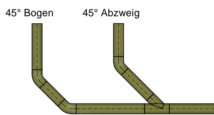
SW Leitung in der Waagerechten
