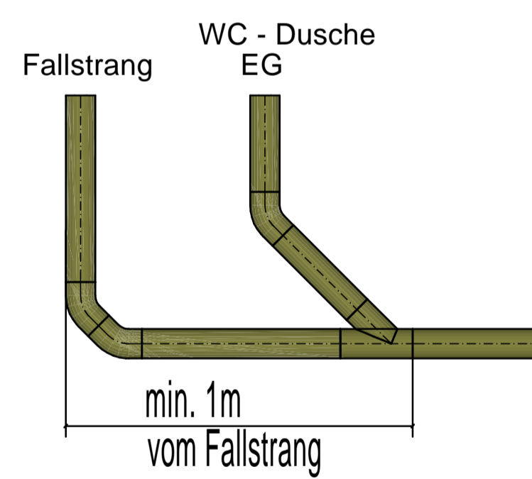
WC - Duschen im KG an die Kellerleitung anschließen
