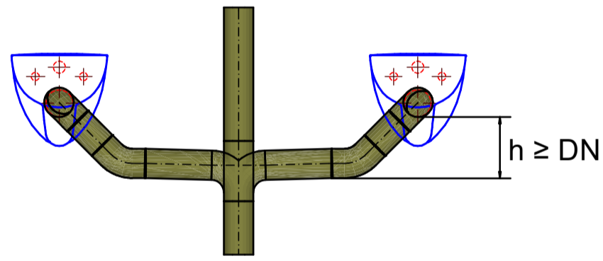
Doppelabzweig 180^\circ mit innenradius
